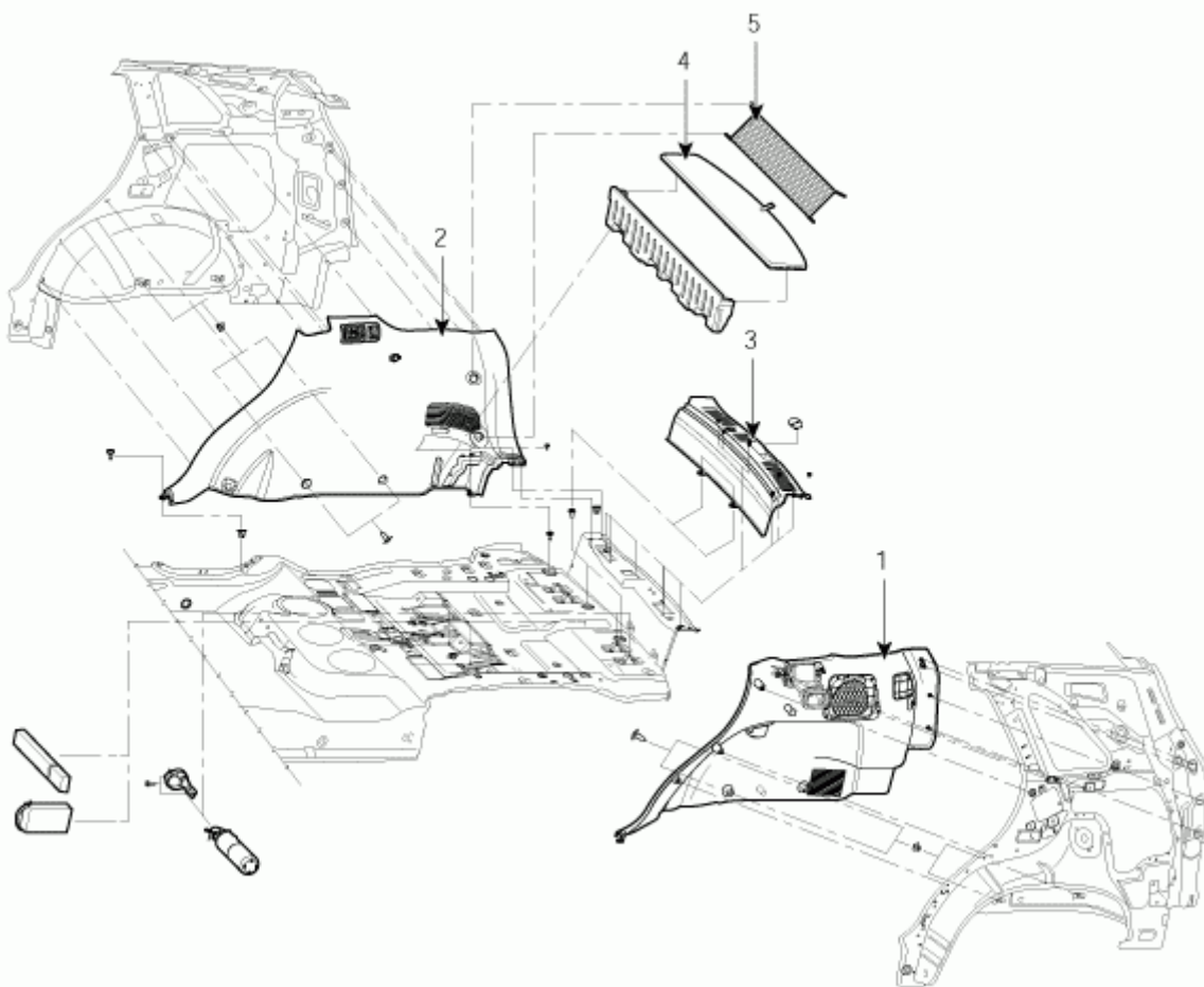
1. 行李箱侧面装饰板(左侧)
